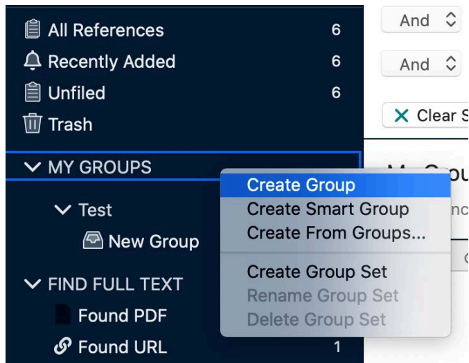
Abbildung 16: Groups anlegen
