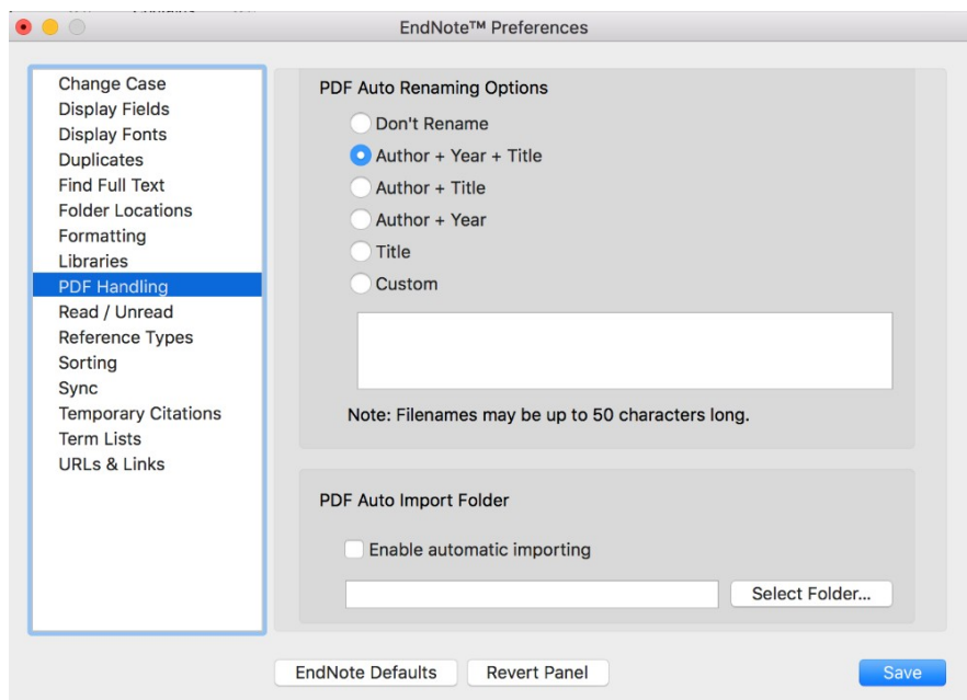
Abbildung 15: PDF Handling
