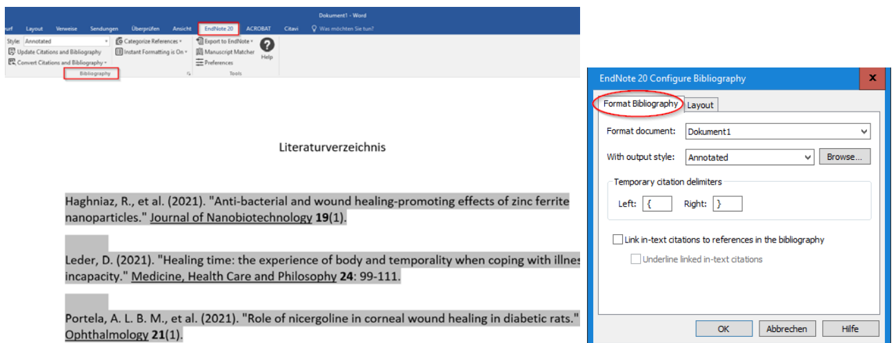
Abbildung 23: Bibliographie formatieren
